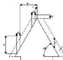
TELHADO A 60°
