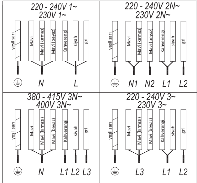
Şekil 2b (7 KABLO)
