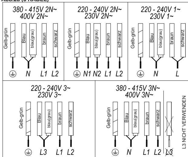
Abb.2a (5 KABEL)
