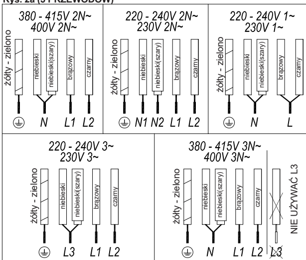
Rys. 2a (5 PRZEWODÓW)
