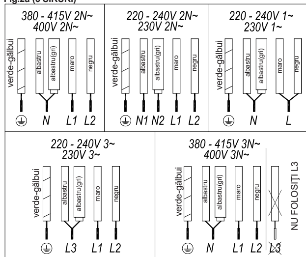
Fig.2a (5 SIRURI)
