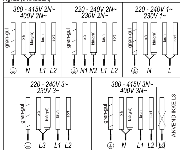
Fig. 2a (5 KABLER)
