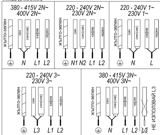
Фиг.2а (5 ЖИЛКИ)
