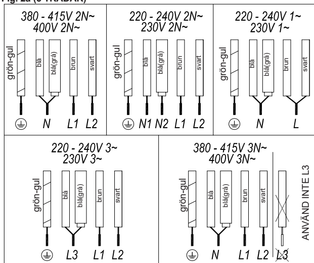
Fig. 2a (5 TRÄDAR)
