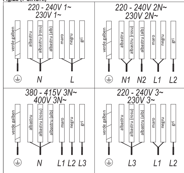
Fig.2b (7 SIRURI)
