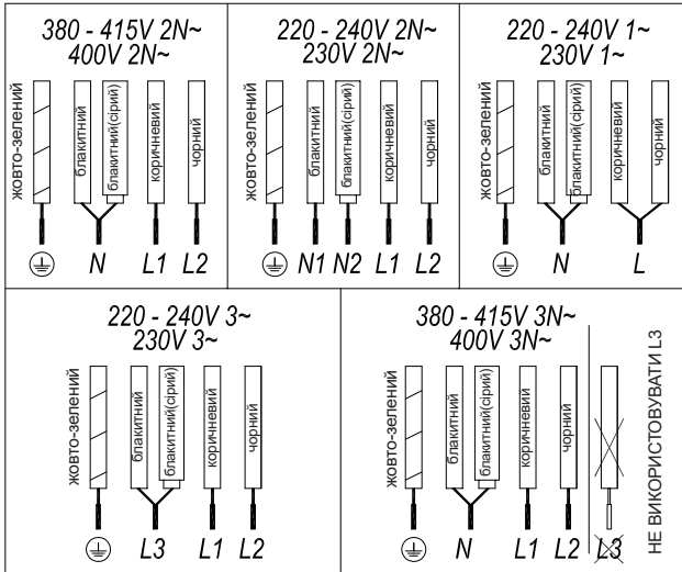
Рис. 2а (5 проводів)
