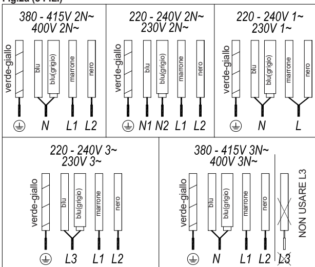
Fig.2a (5 FILI)
